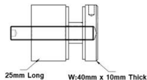
GLH1017-A-Satin GLH1017-A-Mirror W:40mm x L:25mm
